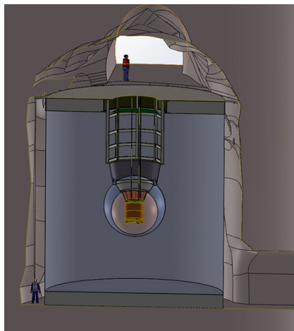
nEXO Experiment
